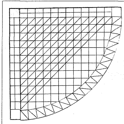
İbnü's-Şâtir'in er-rub'u'l-Alâisi
